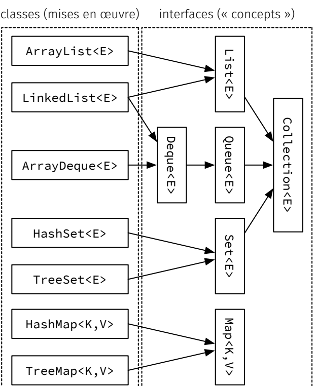
Fig. 1 : Hiérarchie partielle et simplifiée des collections Java
