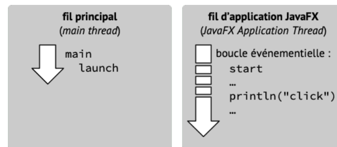
Fig. 4 : Fils d'exécution d'un programme JavaFX simple
