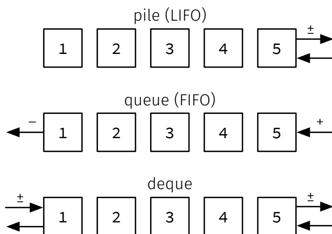
Fig. 2 : Piles, queues et dequeues
