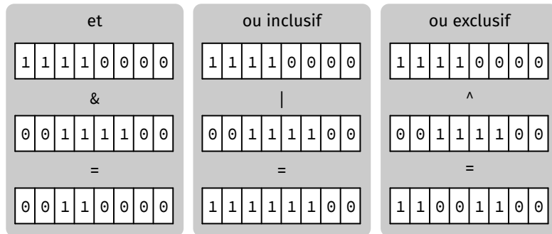
Fig. 2: Exemple des opérateurs bit à bit
