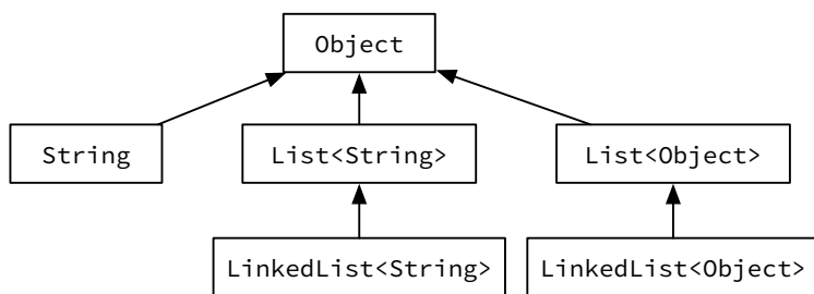
Fig. 2: Absence de sous-typage entre instanciations de List
