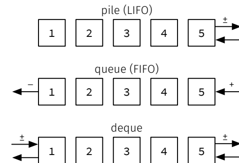
Fig. 2: Piles, queues et dequeues
